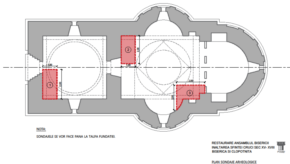
Planul Bisericii Pătrăuți, cu marcarea (roșu) casetelor pentru săpături arheologice
